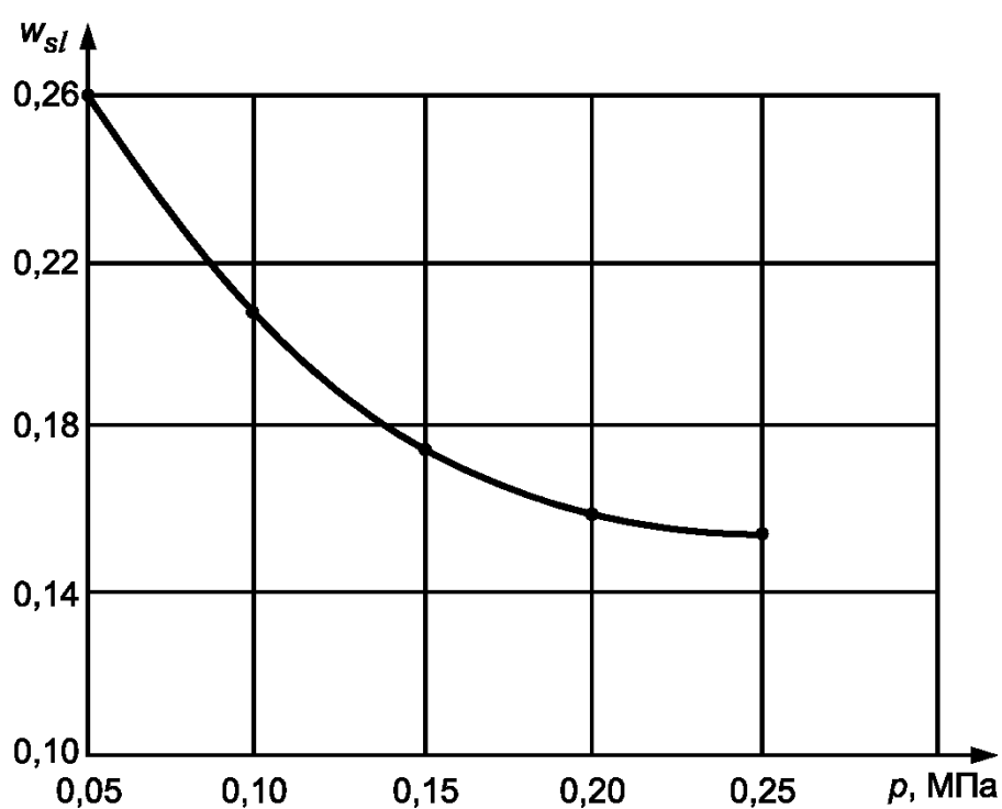
б) График зависимости начальной просадочной влажности w_{sl} от давления \rho
